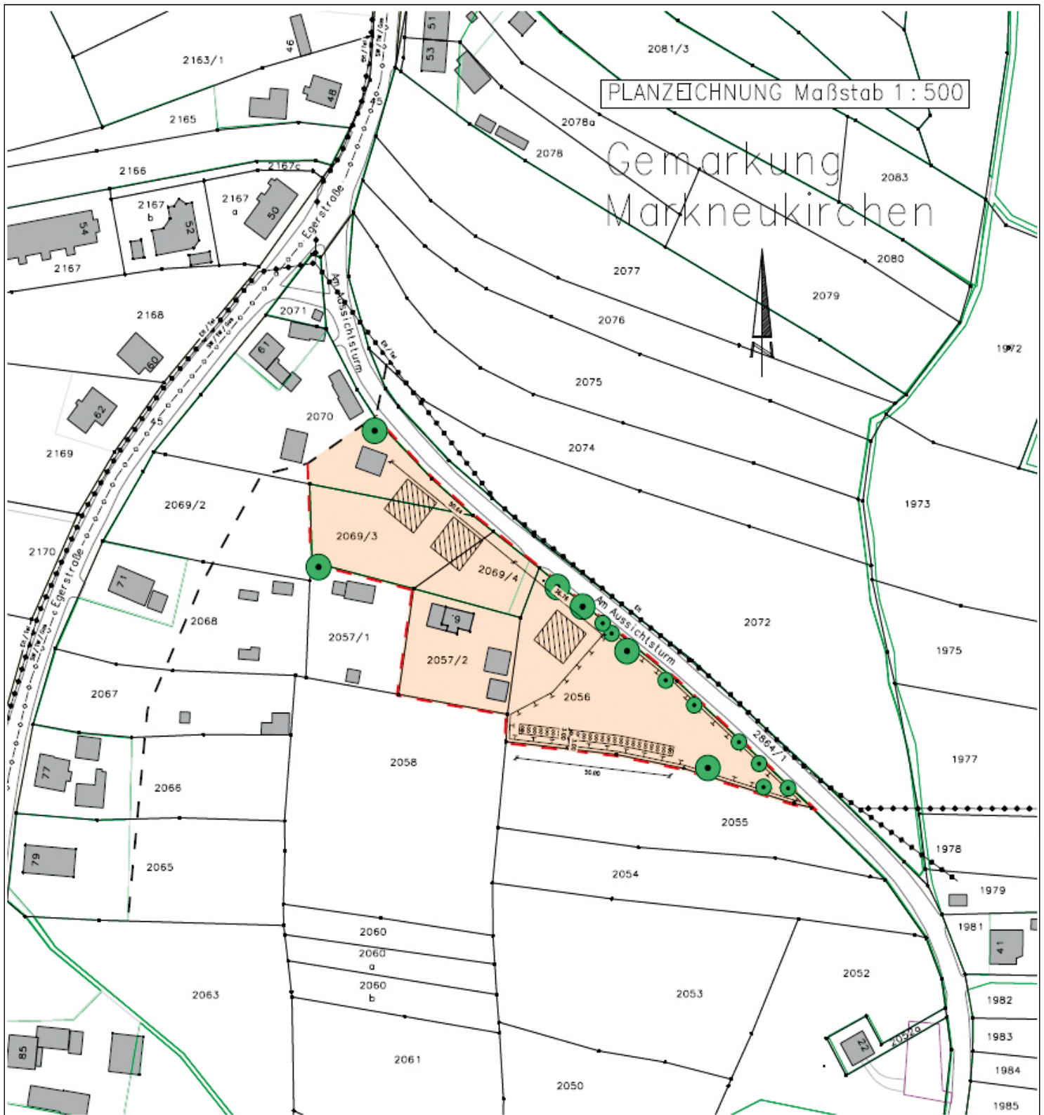
Ausschnitt aus der Planzeichnung der Klarstellungs- und Ergänzungssatzung nach § 34 Abs. 4 Nr. 1 und 3 BauGB „Am Aussichtsturm“ in Markneukirchen, Stand Entwurf 23.05.2022
